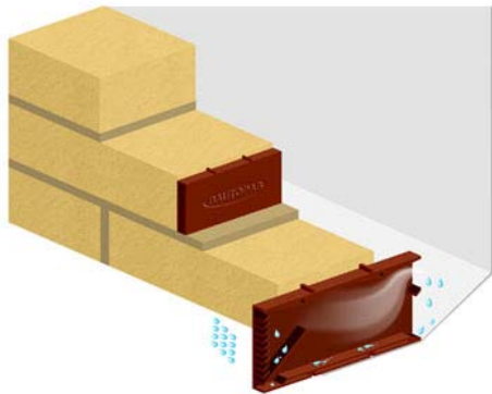
Вентиляция фасада
